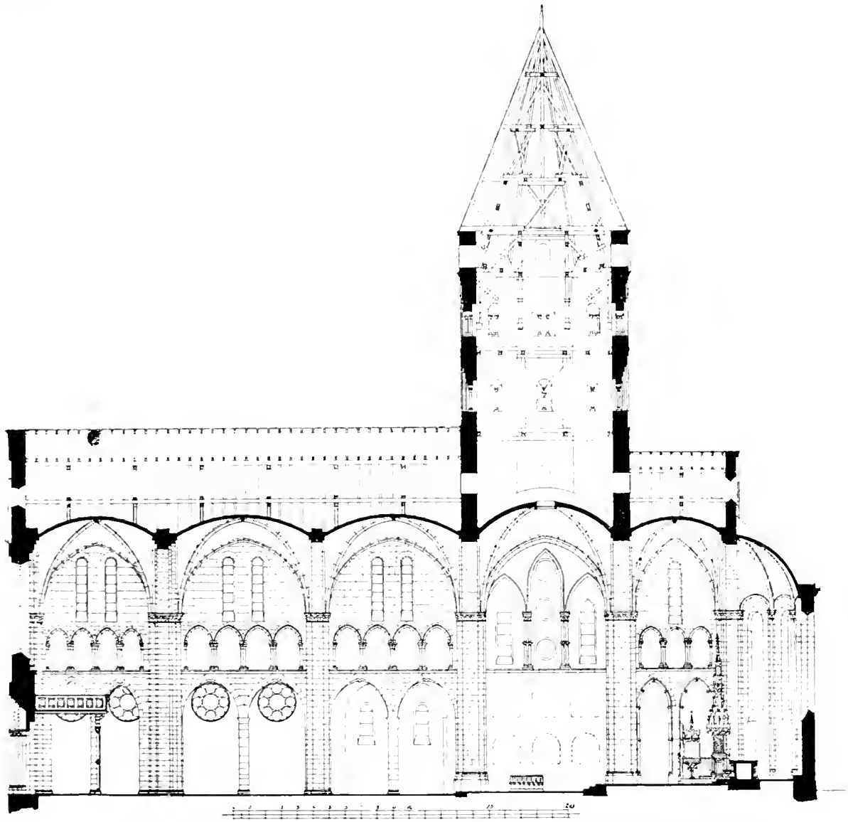
Fig. 37 Gerresheim. Längsschnitt der Stiftskirche.
